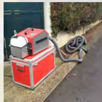
Exemple d'outil de contrôle de conformité de raccordement (appareil à la fumée)
